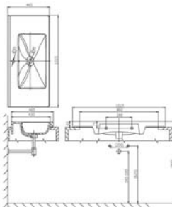
100cm Vessel Basin (1-Hole) Size: 1015 \times 465 \times 175 \text{mm} Material: Vitreous china 100公分柜盆(单孔) 尺寸: 1015 \times 465 \times 175 \text{mm} 材质: 陶瓷
